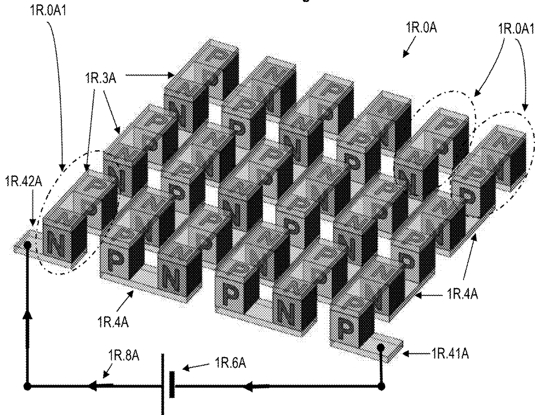
Prior Art Fig. 1r
