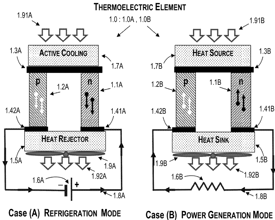
Prior Art Fig. 1p
