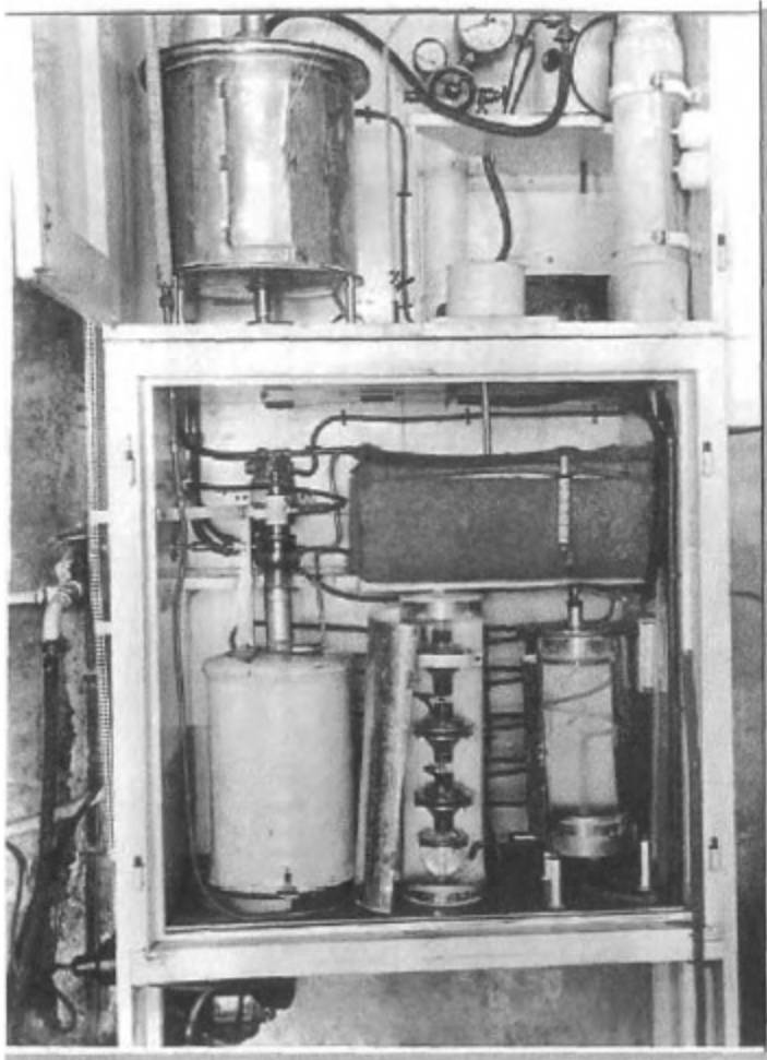
Apparatur zur Herstellung von quellwasserähnlichem Trinkwasser
