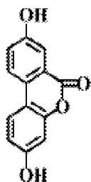
Urolithin A (UA)
